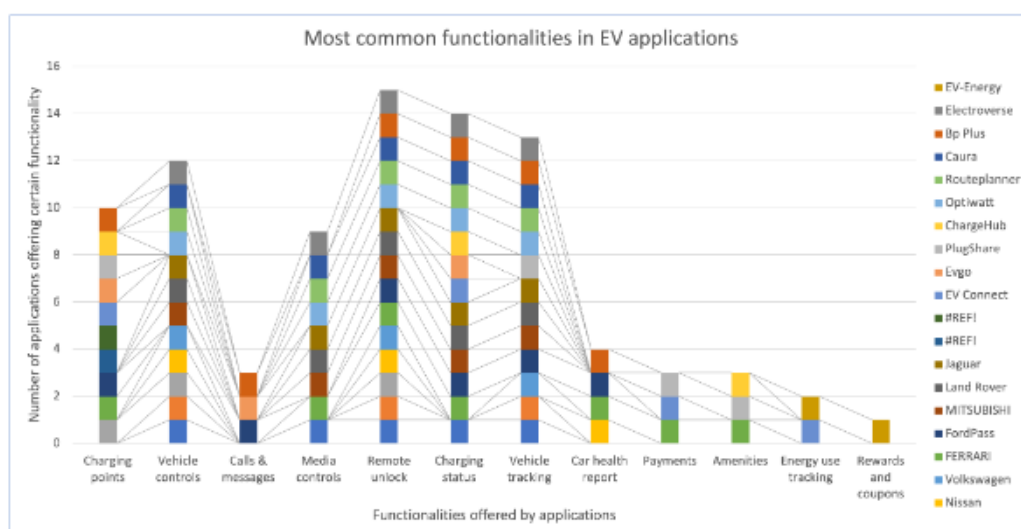
Figura 2: Funcionalidades mais comuns em aplicações EV
